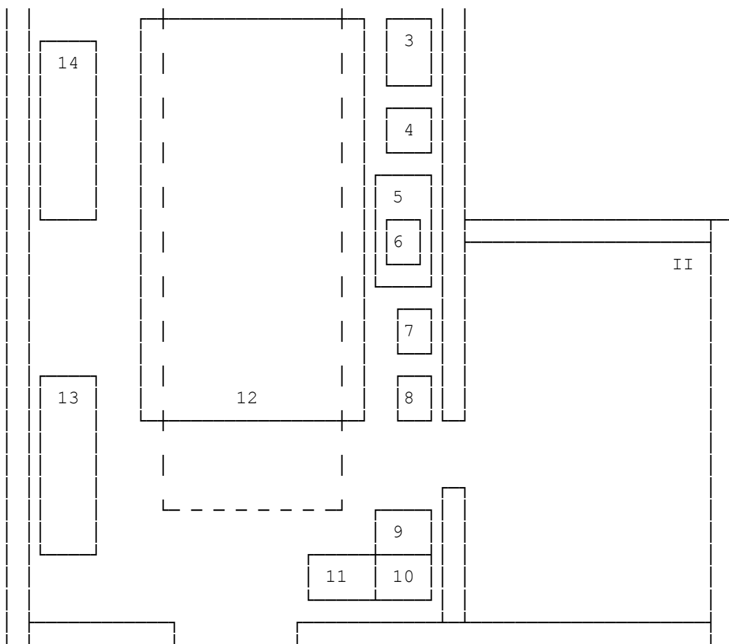
Рис. 5.5. Участок ТО и ТР газобаллонных автомобилей
