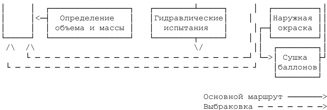
Рис. 10.2. Технологическая схема освидетельствования баллонов
