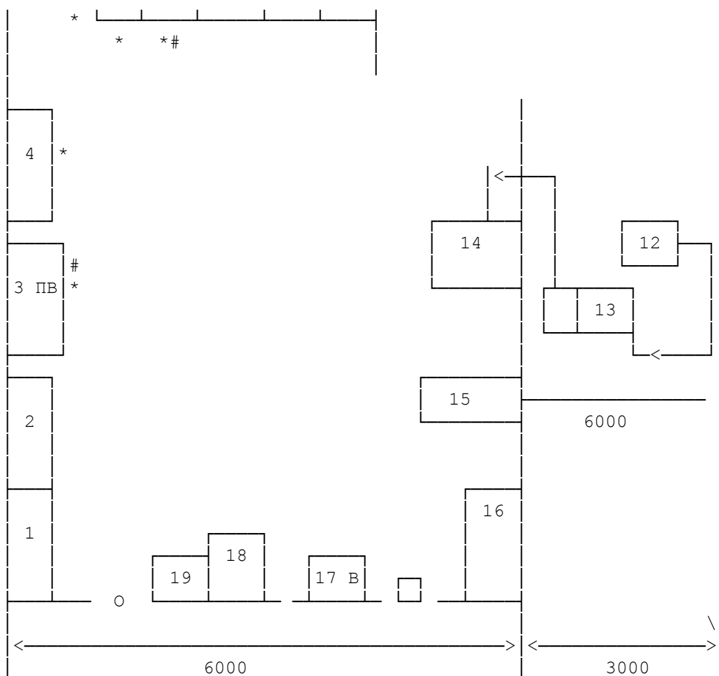
Рис. 5.6. Примерная планировка цеха ТО и ТР газовой аппаратуры в АТП
