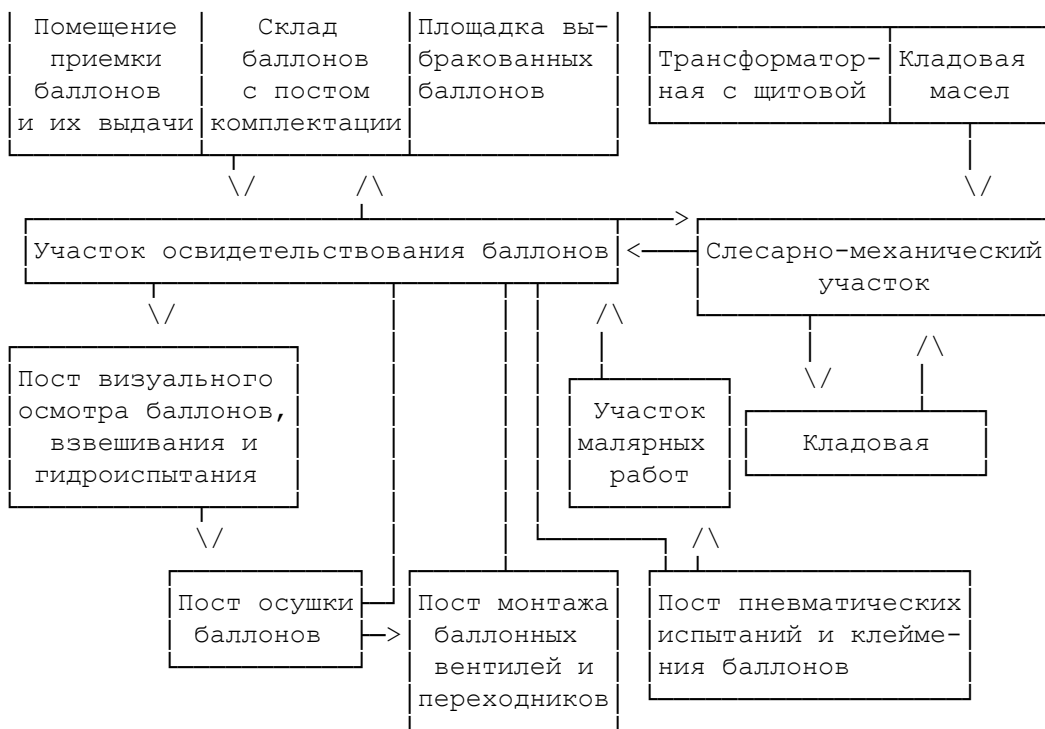
Рис. 10.1. Схема пунктов освидетельствования баллонов
