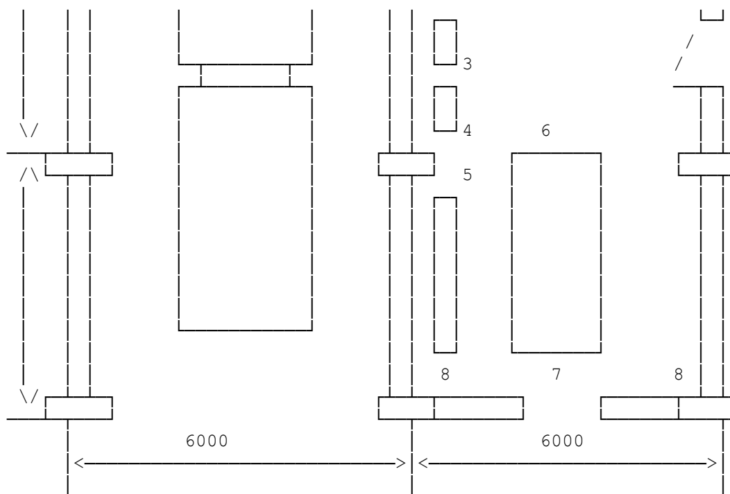
Рис. 5.3. Планировка поста выпуска и аккумулярования газа и дегазации баллонов
