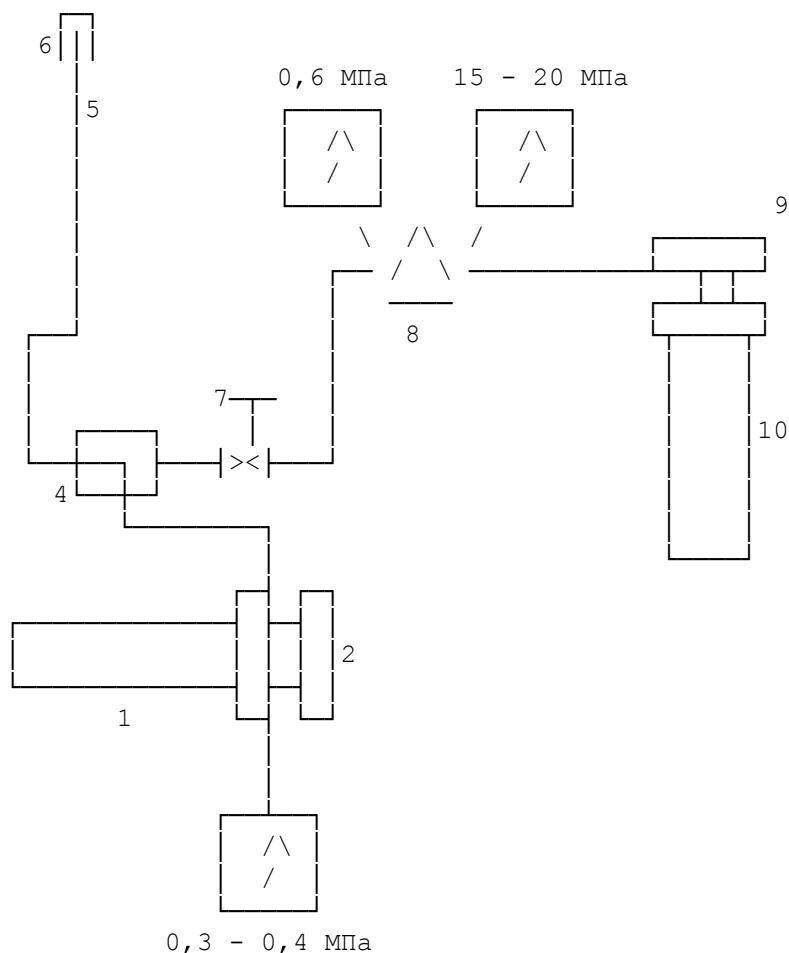
Рис. 5.4. Схема пневматической установки по выпуску газа и дегазации газовых баллонов на автомобиле в условиях АТП
