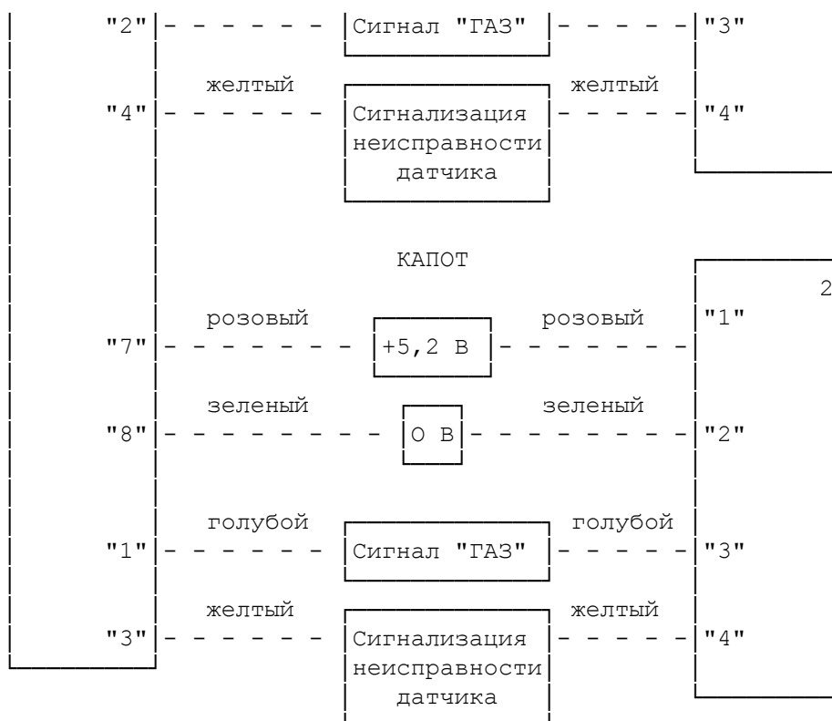
Рис. 7.7. Схема соединений сигнализатора утечки газа (СУГ) на автомобиле ГАЗ-3302 "Газель": 1 - блок питания и индикации; 2 - датчики
