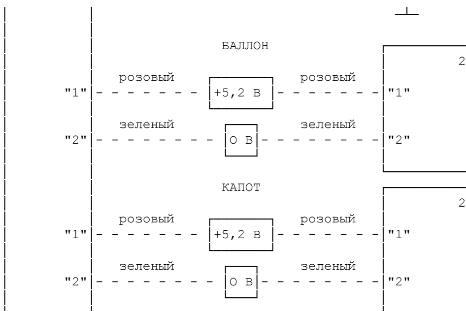
Рис. 7.3. Схема соединений сигнализатора утечки газа (СУГ) на автомобиле Волга: 1 - блок питания и индикации; 2 - датчики
